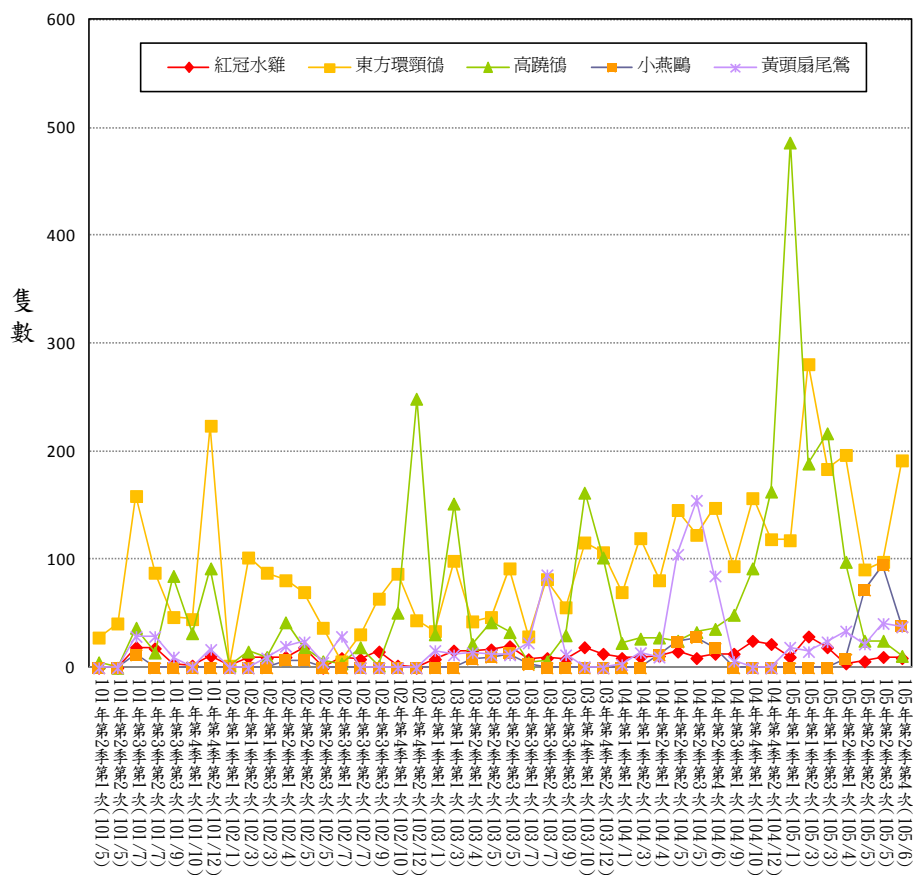
附圖 B-1 通苑風場指標生物歷年各季比較圖
